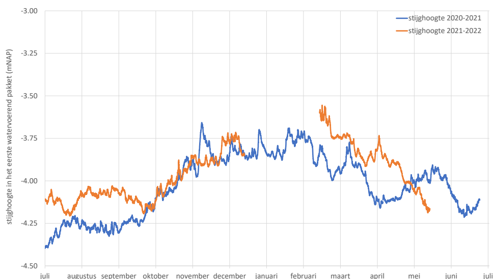
Figuur 14 B37E0312 aan het Baden Powellpad. De stijghoogte in het najaar van 2020 en 2021 zijn om en nabij aan elkaar gelijk. Door een fout in de apparatuur zijn de metingen tussen half december en half februari verloren gegaan. Nu in mei 2022 zijn de metingen weer om en nabij aan elkaar gelijk.
