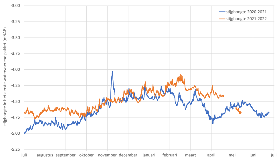
Figuur 13 B37E3473 in de Doelenstraat. De stijghoogte in 2020-2021 en 2021-2022 zijn tot eind januari om en nabij aan elkaar gelijk. Door het uitzetten van de bronnen op het DSM terrein is de stijghoogte na januari 2022 hoger dan na januari 2021.
