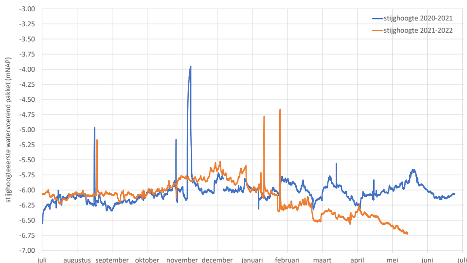
Figuur 11 B37E3507 aan de Foreestweg. De stijghoogte in 2020-2021 en 2021-2022 zijn tot eind januari om en nabij aan elkaar gelijk. Door het uitzetten van de bronnen op het DSM terrein is de stijghoogte na januari 2022 lager dan na januari 2021.
