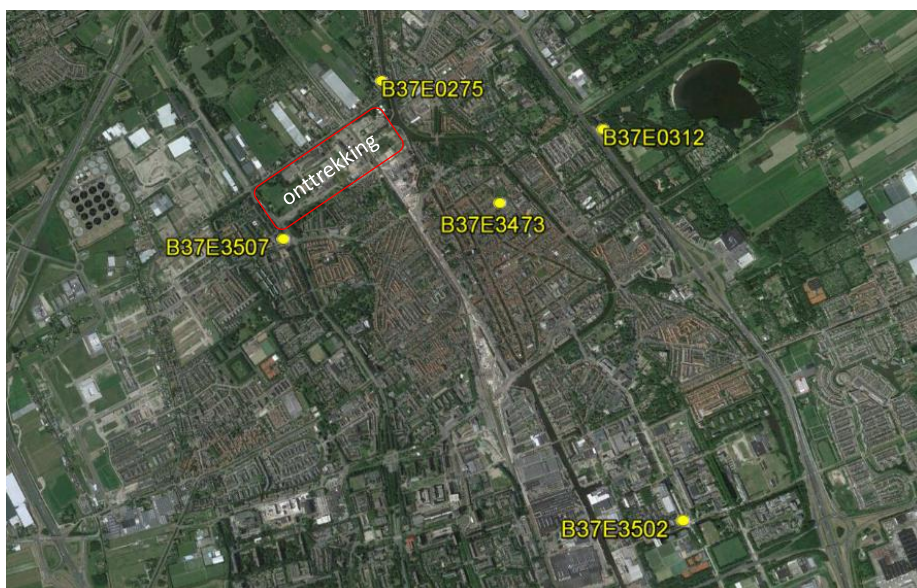
Figuur 5 locaties van de 5 peilbuizen uit het eerste watervoerend pakket
