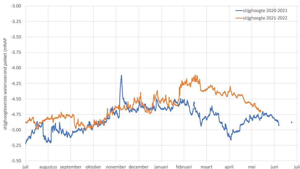
Figuur 12 B37E0275 aan 't Haantje. De stijghoogte in 2020-2021 en 2021-2022 zijn tot eind januari om en nabij aan elkaar gelijk. Door het uitzetten van de bronnen op het DSM terrein is de stijghoogte na januari 2022 hoger dan na januari 2021. Inmiddels is in mei 2022 de stijghoogte weer om en nabij gelijk aan de stijghoogte van mei 2021.
