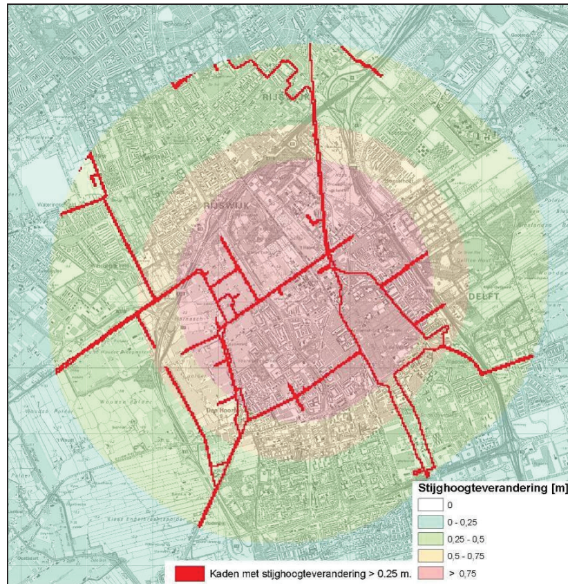
Figuur 5.3: Kaden met stijghoogteverandering > 0,25 m bij een winning van 1000 \text{ m}^3/\text{uur}
